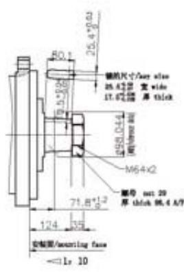
STFC HD200-T72
