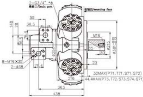
STFC200-P71
