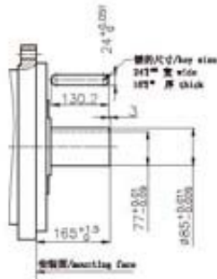
STFC200-T71
