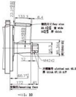
STFC200-T71
