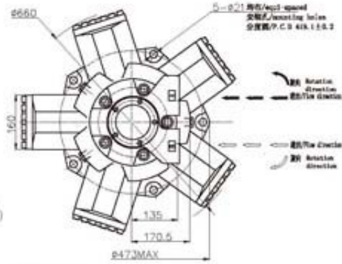
STFC HD200-★P73
