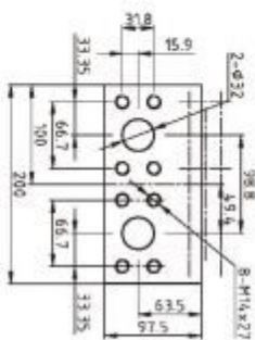
A/C 接口/Conn.A/C
